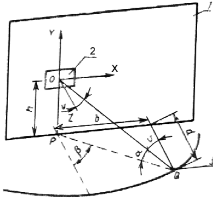
1 - наружная стена; 2 - испытываемый образец; 3 - громкоговоритель
